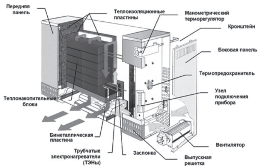
Рисунок А.6 – Схема работы аккумуляционного комнатного обогревателя
