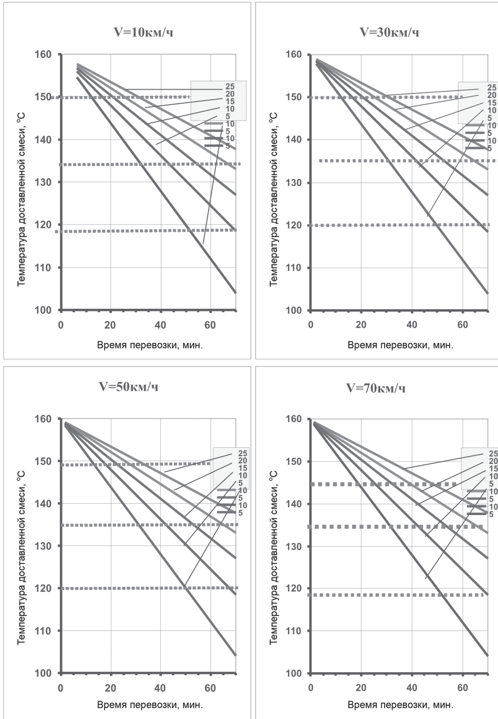
Рисунок В.1 – Время перевозки горячей асфальтобетонной смеси в автомобилях самосвалах (при температуре отгрузки t_{\text{нач}} = 160 \text{ °C} )
