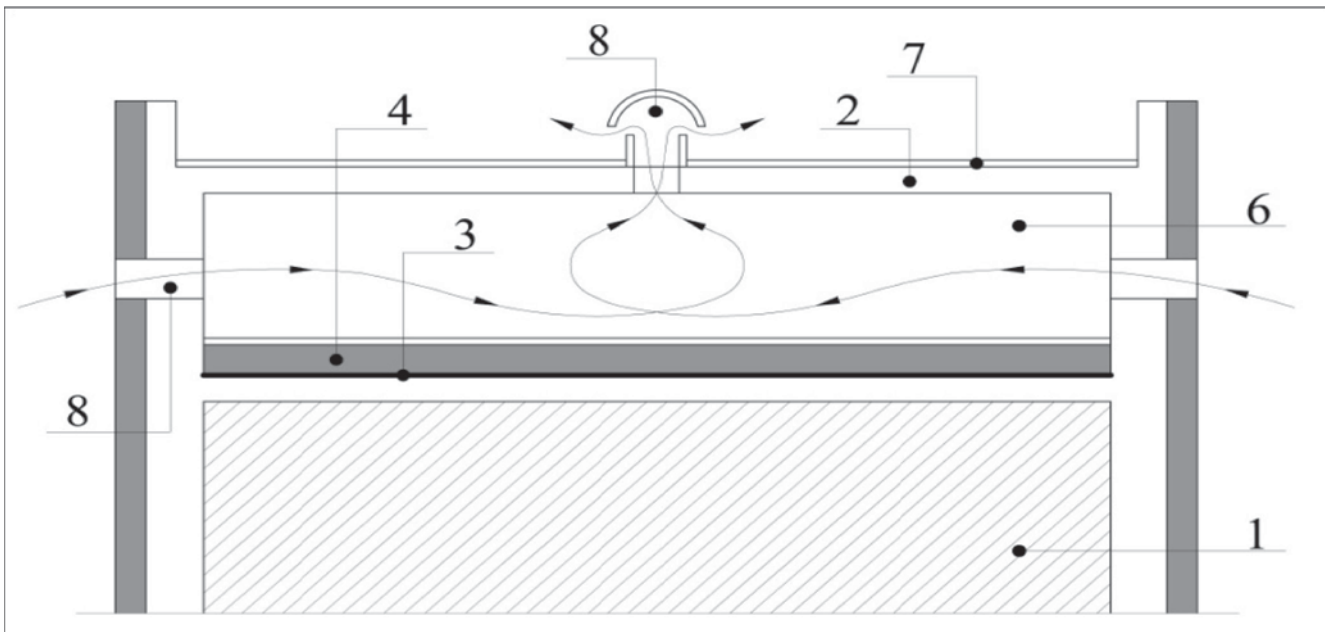
б – утепленная чердачная плоская крыша
