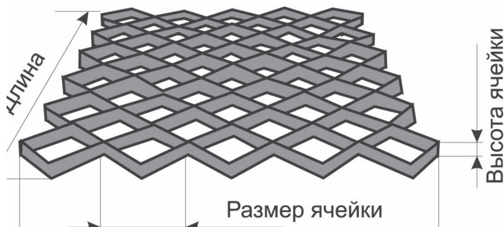
б) схема растяжения объемной георешетки
