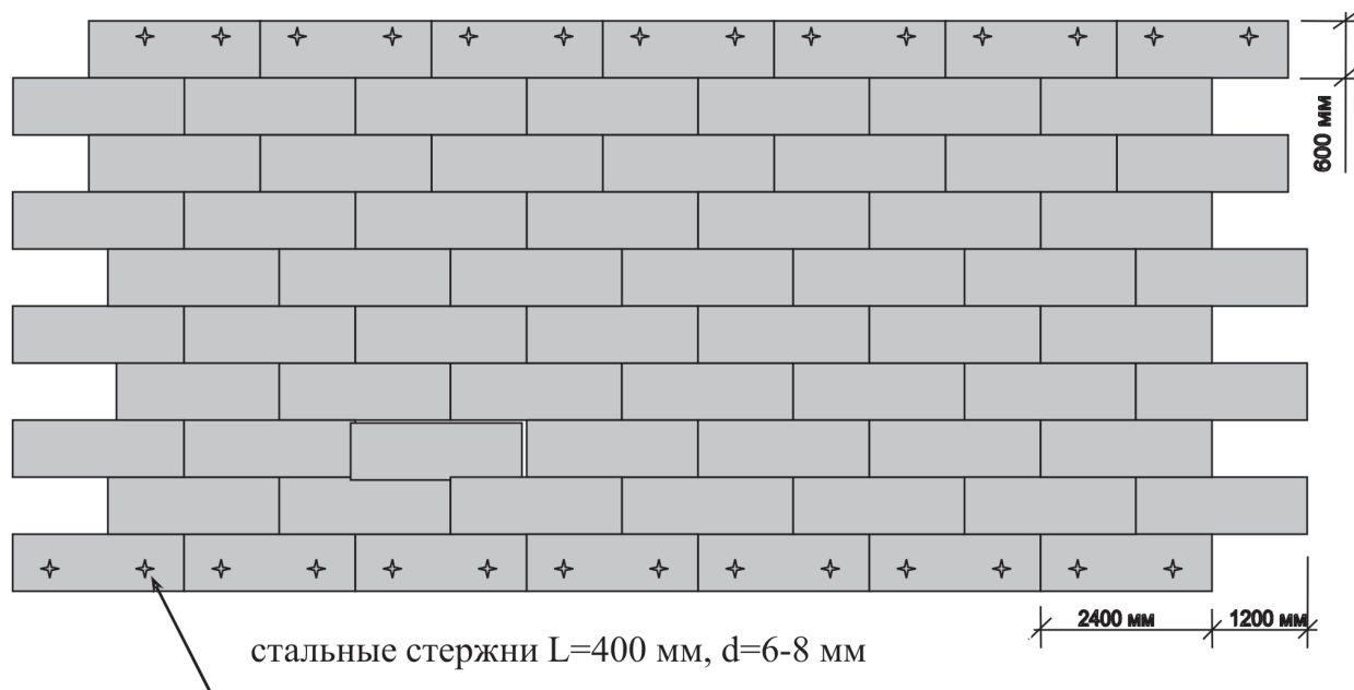
Рисунок 5 – Раскладка вспененных геоплит в теплоизоляционном слое
